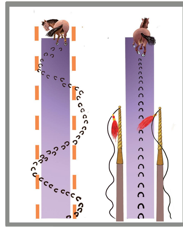
约束力
